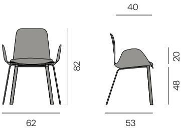
PEC mit festem Gestell, mit Armlehne, mit Kissen PEC with fixed base, with armrest, with cushion
