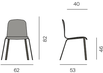
PEC mit festem Gestell PEC with fixed base
