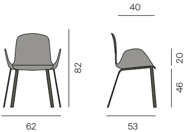
PEC mit festem Gestell, mit Armlehne PEC with fixed base, with armrest
