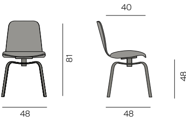
PEC mit drehbarem Gestell, mit Kissen PEC with revolving base, with cushion
