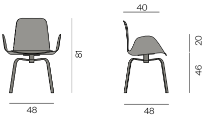
PEC mit drehbarem Gestell, mit Armlehne PEC with revolving base, with armrest
