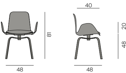
PEC mit drehbarem Gestell, mit Armlehne, mit Kissen PEC with revolving base, with armrest, with cushion
