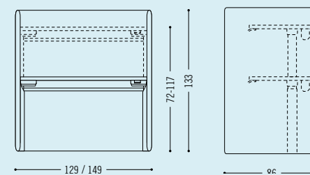
Tischplatte elektrisch höhenverstellbar/tabletop electrically height adjustable
