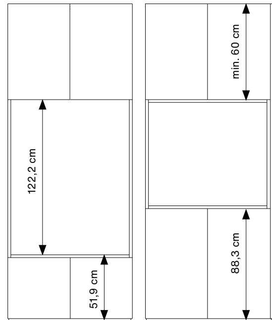
Nischenelement / Niche element
