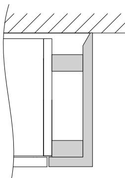
D. mit Außenwange / D. with infill panel
