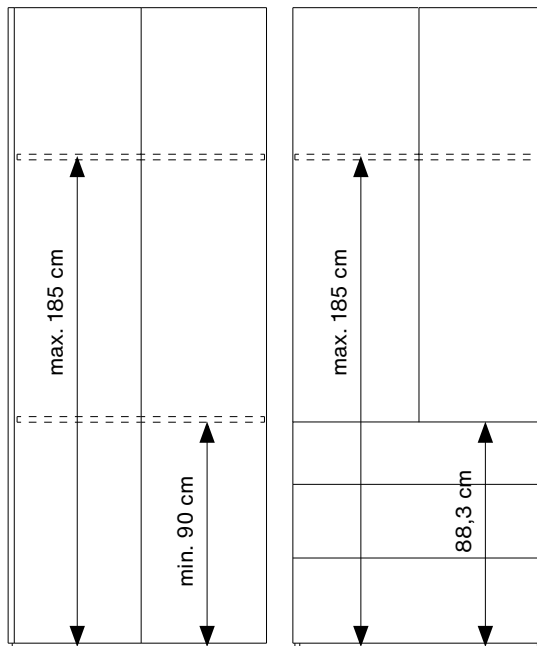
Schränkelement / Cupboard element
