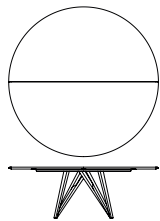
2759 Ø 220 H 75
